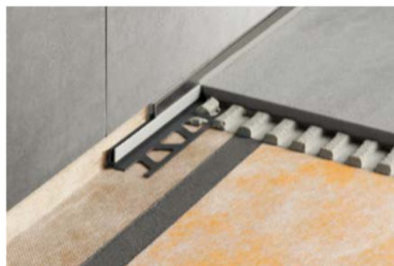
Schlüter-SHOWERPROFILE-S Einbau an der Wand
